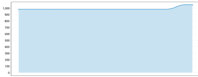
Bugs
